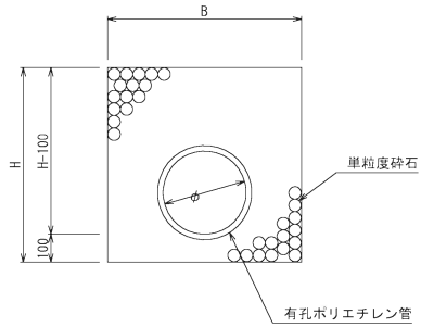
暗渠工 S=1:10
